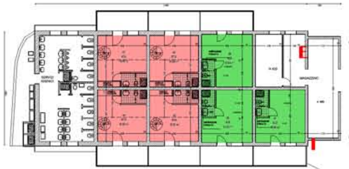
PIANO TERRA EDIFICIO (C) SCALA 1:200
